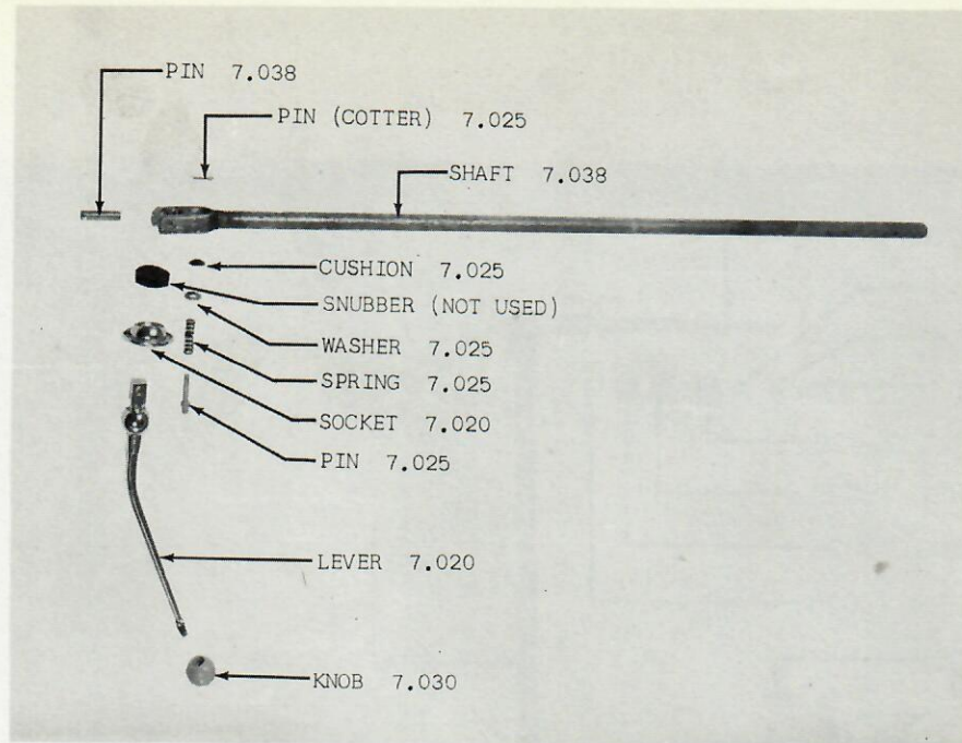
GROUP 7 - FIG. 1 - GEAR SHIFT LINKAGE (UPPER) 01 (LAT)
